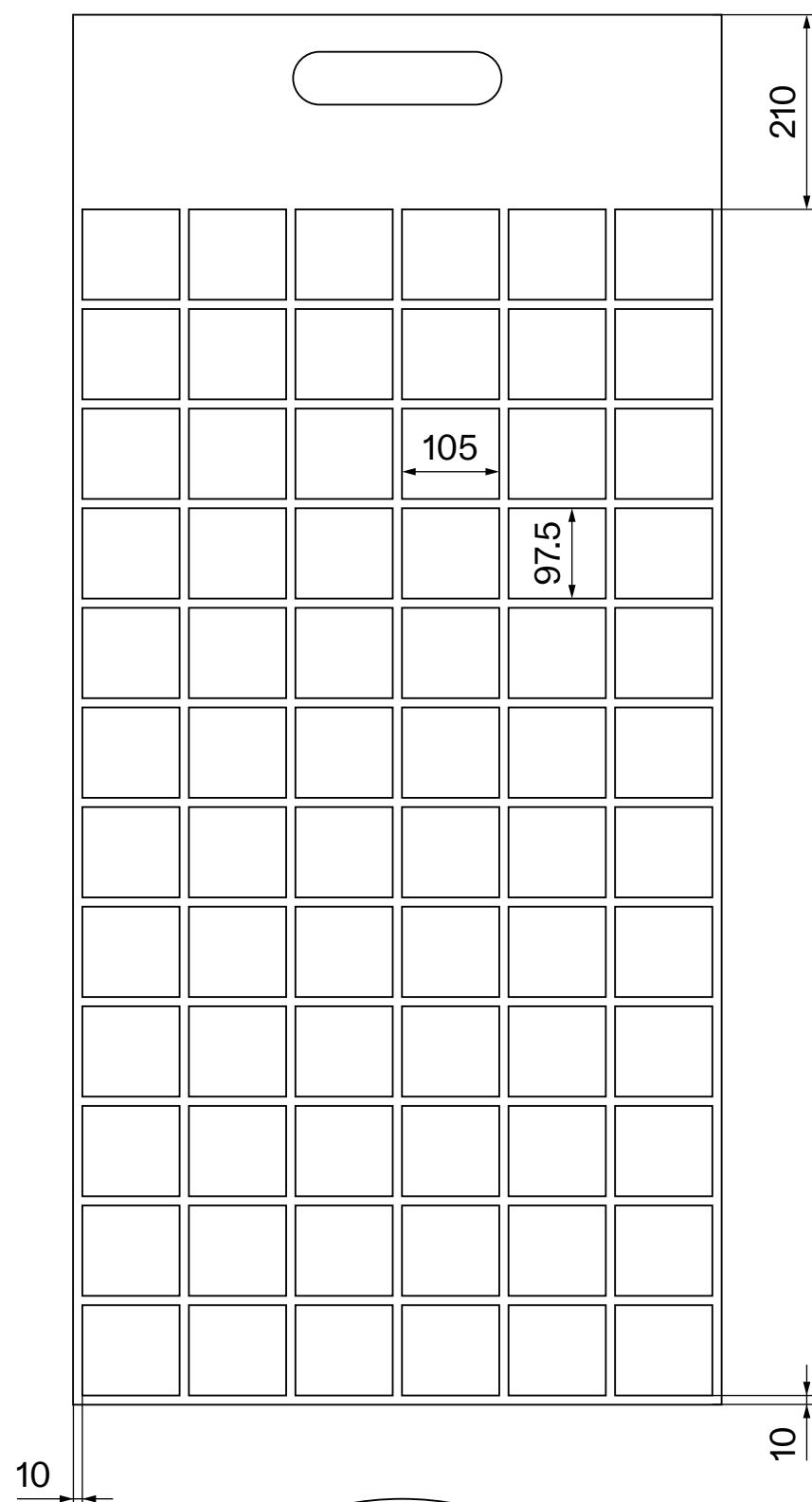
Detail A-A
