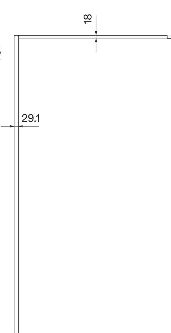
Section A-A
